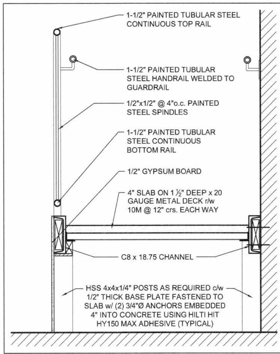
7 RAMP DETAIL SCALE: 1" = 1'-0"
