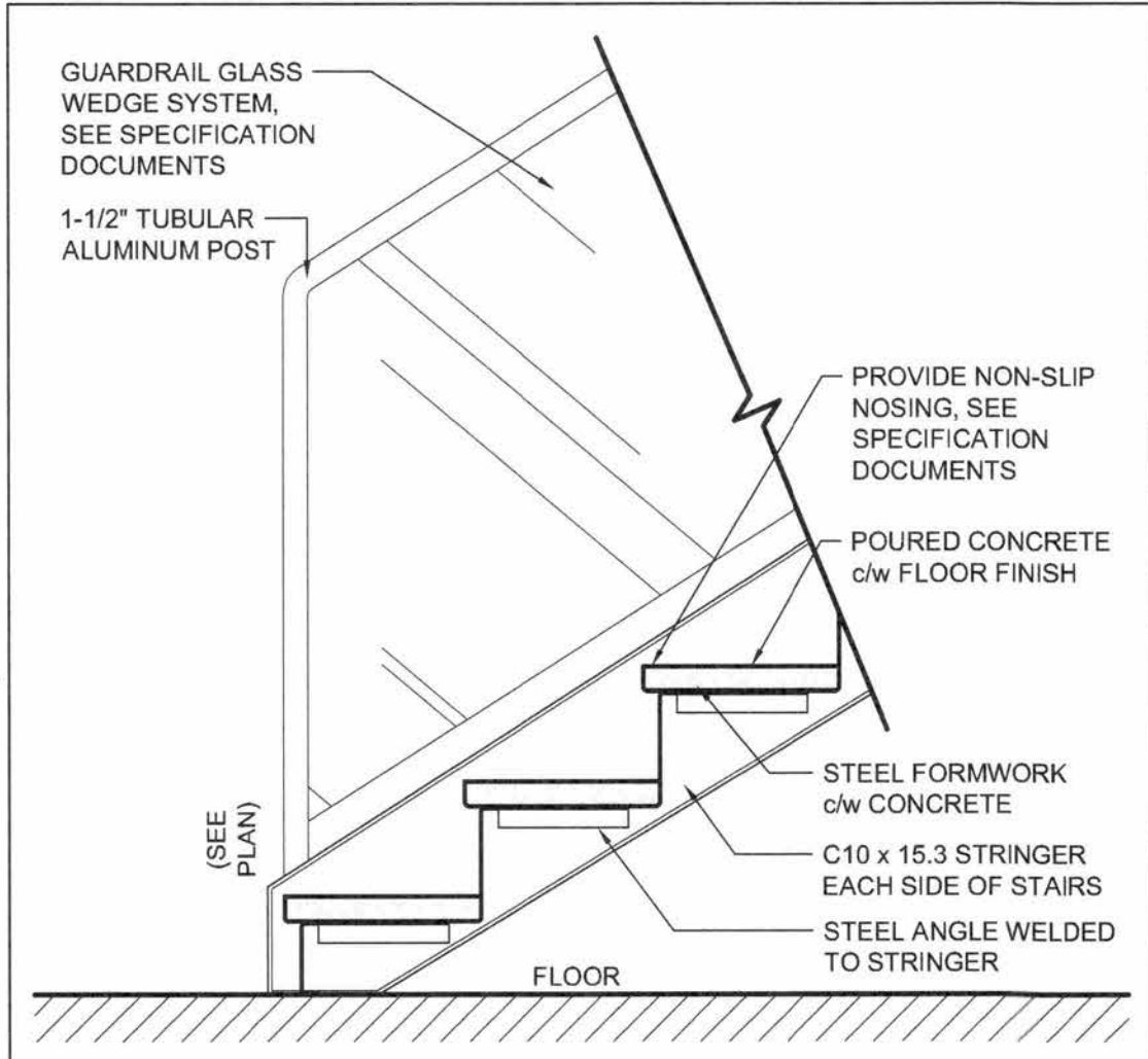
4 STAIR DETAILS SCALE: 1" = 1'-0"
