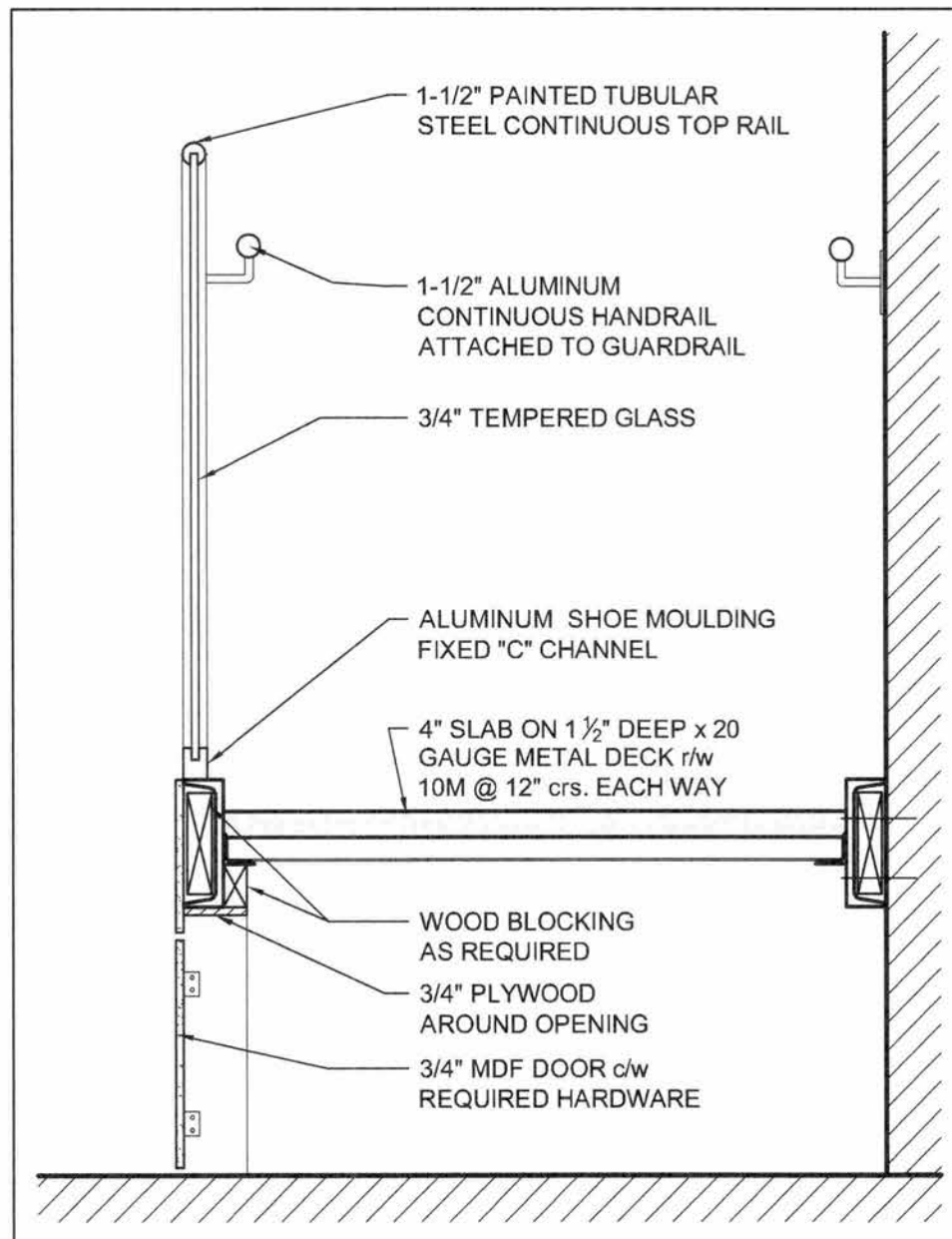
5 RAMP DETAIL SCALE: 1" = 1'-0"
