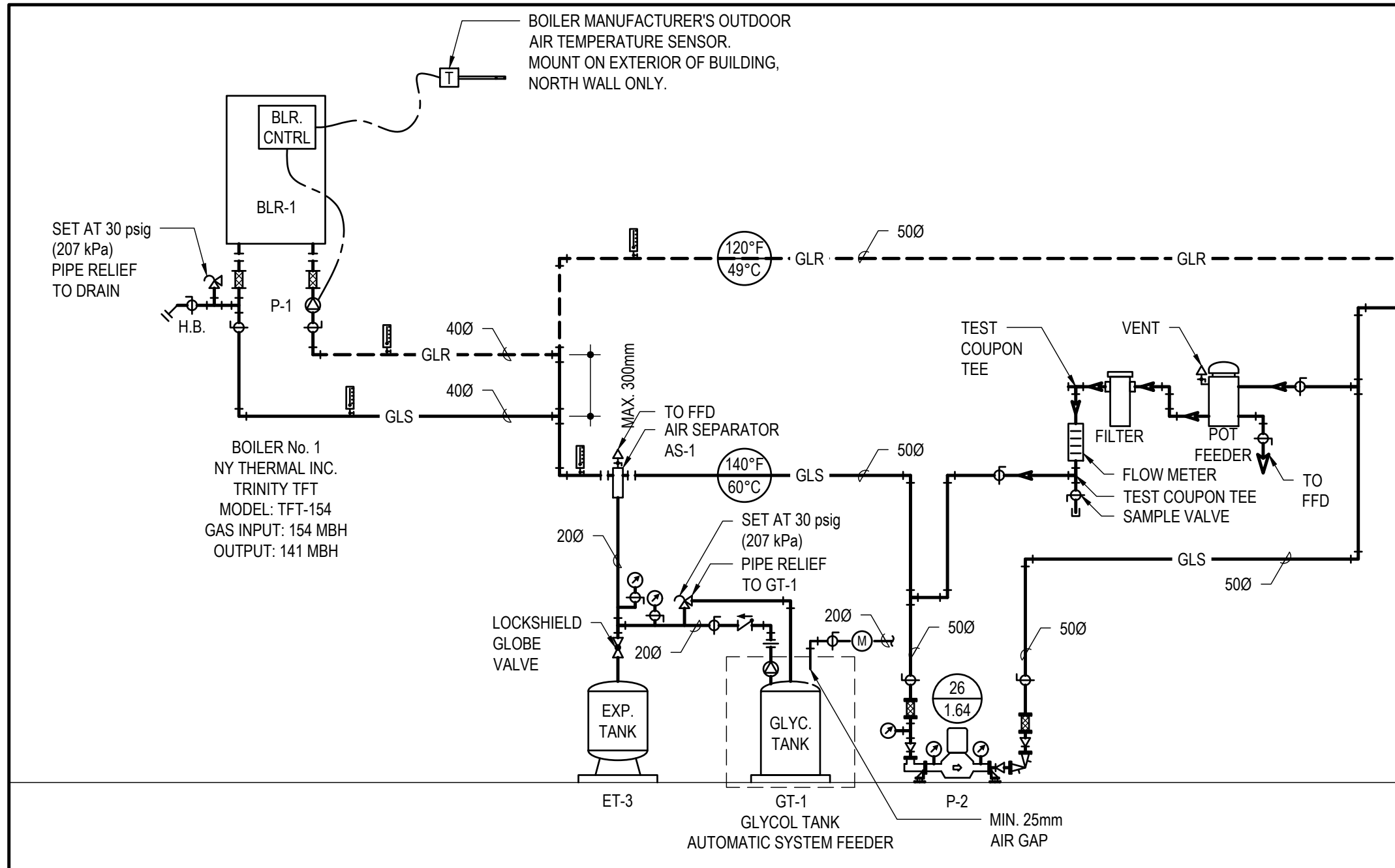
1 HYDRONIC HEATING SCHEMATIC M301 SCALE: N.T.S.
